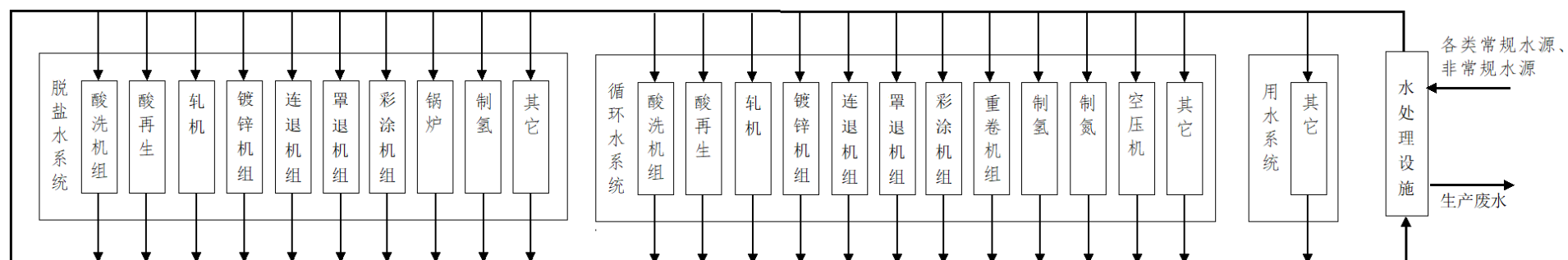
图A.1 冷轧工序用水平衡图
