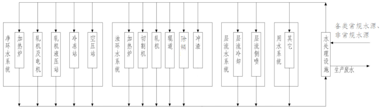
图 1 热轧工序用水平衡图
